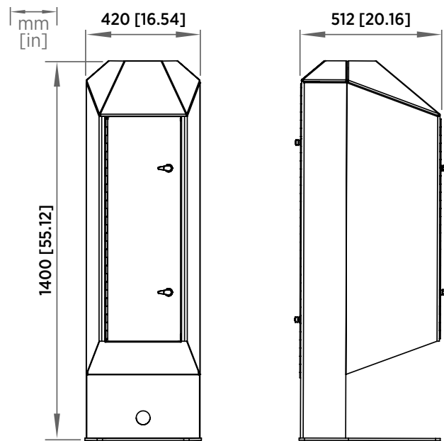
CL61 dimensions
